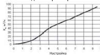
Расходная характеристика
